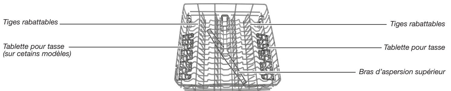
PANIER SUPÉRIEUR
